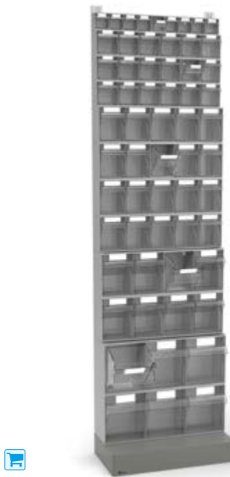
SCAFFALE CON 61 CASSETTI VISUAL BOX DIM. (mm): L=604 P=322 H=2100
