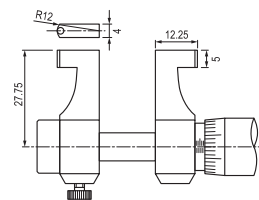
Contatti campo di misura 25-50 mm
