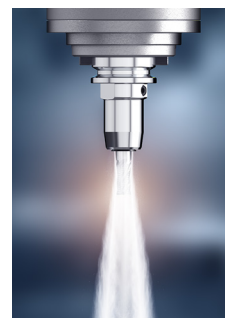
Boccole di riduzione 05FHC...L1 con canali per adduzione del refrigerante periferici per utensili privi di fori per l'adduzione del refrigerante interna
